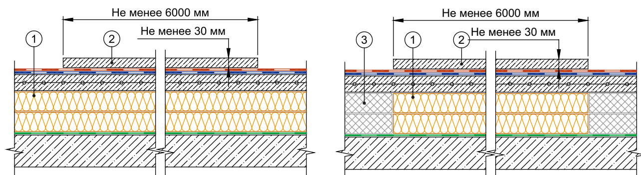
Рис. 4.1. Варианты устройства противопожарных рассечек: 1 – утеплитель НГ и Г1; 2 – монолитная стяжка; 3 – утеплитель ГЗ-Г4
