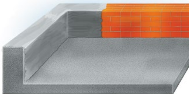
Рис. 3.14. Оштукатуривание вертикальной поверхности
