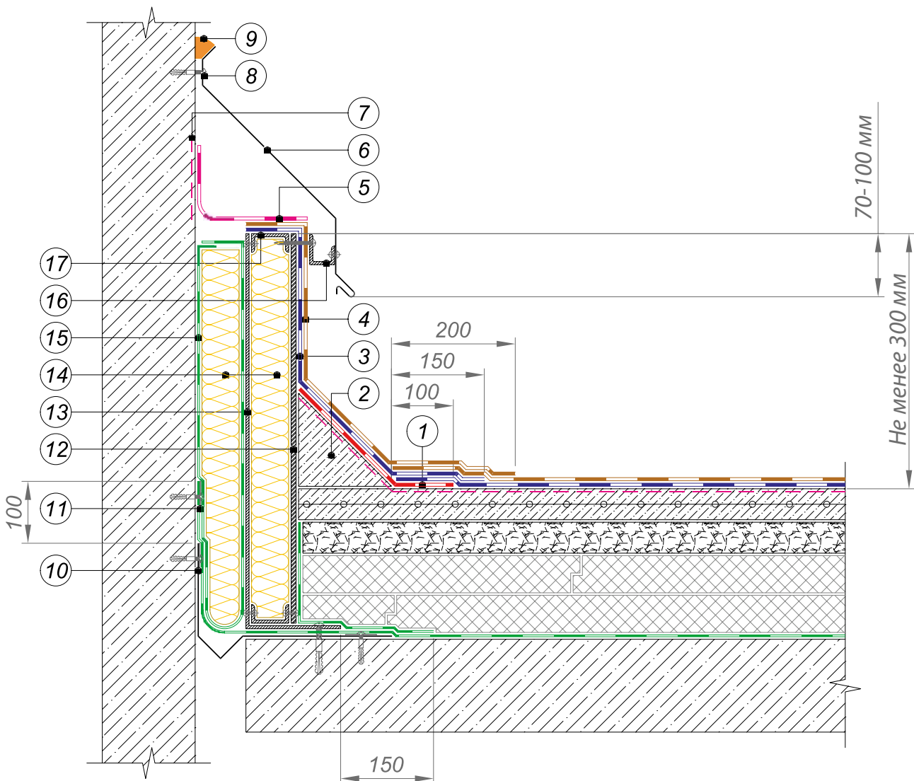
Рис. 3.59. Тип Д. Деформационный шов в месте сопряжения двух разновысоких частей здания: 1 – слой усиления; 2 – переходный бортик; 3 – нижний слой водоизоляционного ковра – Техноэласт ЭПП; 4 – верхний слой водоизоляционного ковра; 5 – бесшовный битумно-полимерный материал Техноэласт ФЛЕКС; 6 – фартук из оцинкованной стали; 7 – праймер битумный ТЕХНОНИКОЛЬ № 01; 8 – крепить саморезами с шагом 200 мм; 9 – мастика ТЕХНОНИКОЛЬ № 71; 10 – компенсатор из оцинкованной стали крепить с фартуком механически; 11 – материал наплавить на вертикальную поверхность и закрепить механически саморезами с шайбой диаметром 50 мм; 12 – хризотилцементные плоские листы (цементно-стружечные плиты марки ЦСП-1); 13 – Профиль из оцинкованной стали толщиной не менее 3 мм; 14 – Минераловатный утеплитель; 15 – Пароизоляционный материал для фиксации утеплителя; 16 – Компенсатор из оцинкованной стали крепить с фартуком механически; 17 – Профиль из оцинкованной стали крепить заклепками
