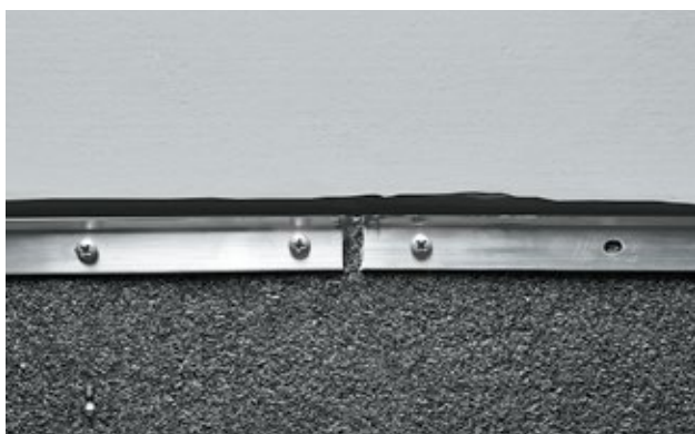
Рис. 3.21. Зазор между краевыми рейками
