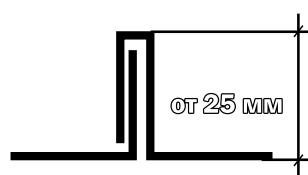
Рис. 3.27. Одинарный стоячий фланец
