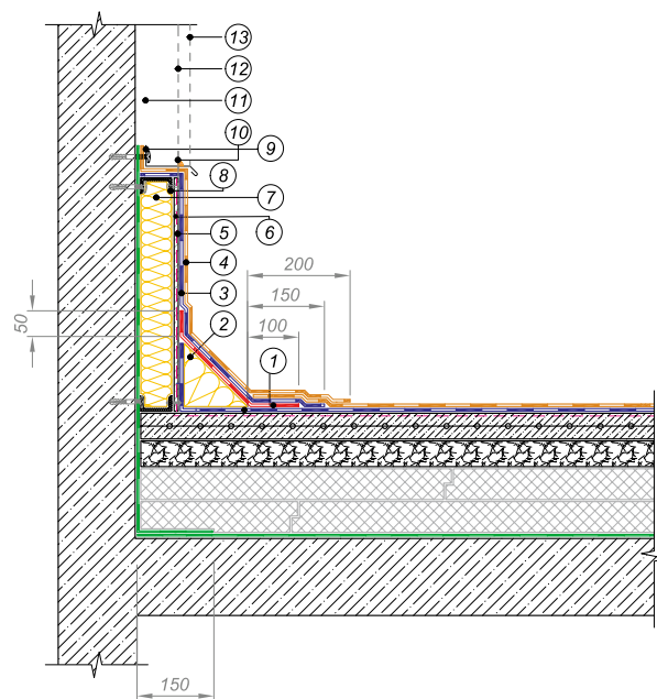
Рис. 3.7. Заведение пароизоляционного слоя к утепленным вертикальным конструкциям
