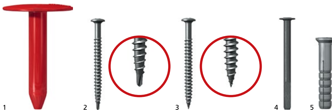
Рис. 3.40. Крепежные элементы при фиксации водоизоляционного ковра через теплоизоляционный слой 1 – Телескопический крепеж; 2 – Сверлоконечный саморез ТехноНИКОЛЬ диаметром 4,8 мм; 3 – Остроконечный винт ТехноНИКОЛЬ диаметром 4,8 мм; 4 – Стальной забивной анкер; 5 – Полиамидная анкерная гильза
